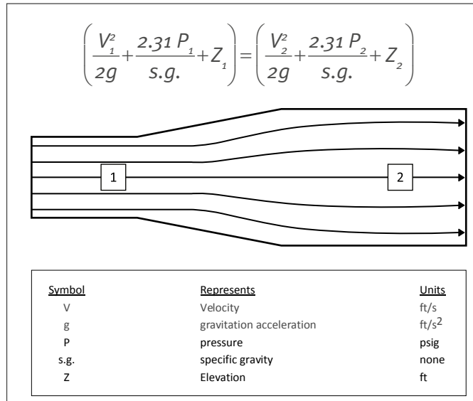
Fig. 12.7. Bernoulli’s Law
