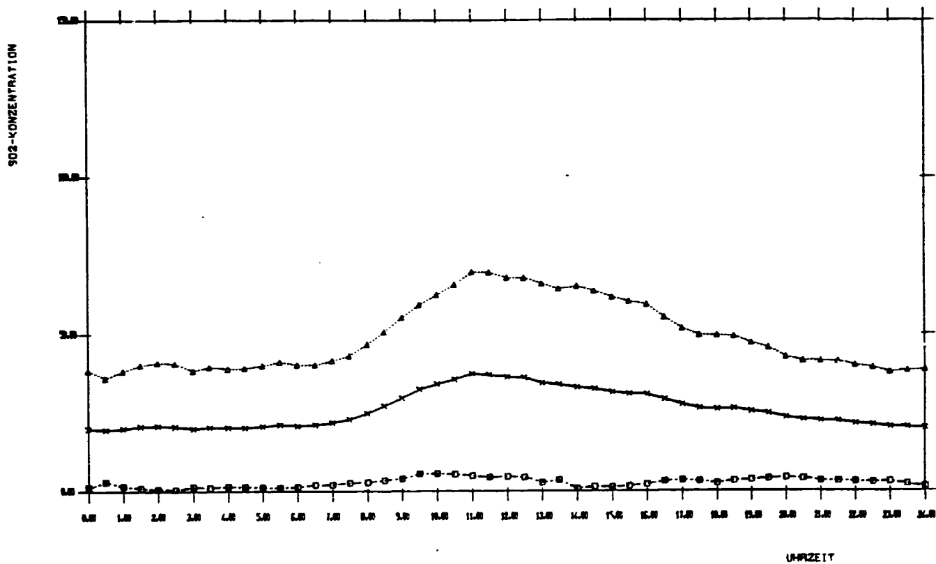
ABB MITTLERER TAGESGANG DER SO 2 -KONZENTRATION IN 10 -3 MG/M 3 IN TRAISNAUER
