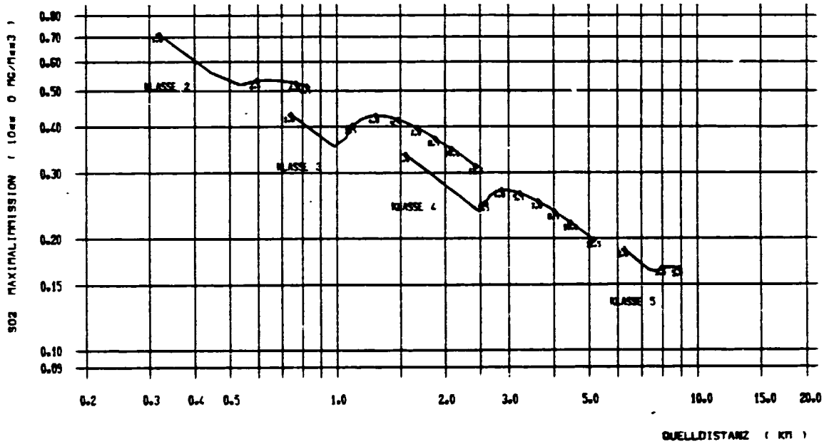
ABB. MAXIMALIMMISSION IN ABHÄNGIGKEIT VON DER WINDGESCHW. > 1.0 M/S
