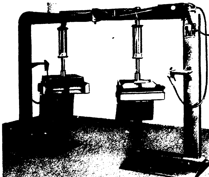
Figura 45. Prensas de asientos
