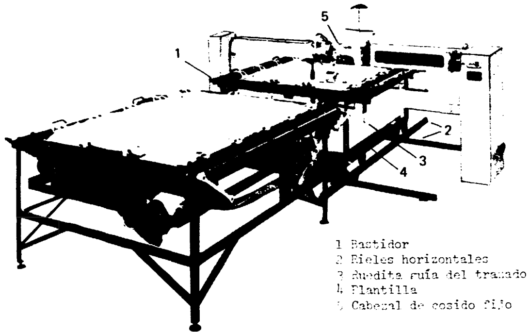
Cabecial simple
