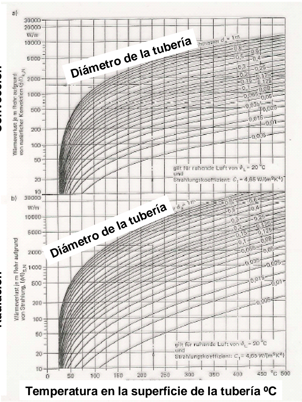
Gráfico 7. Determinación de las pérdidas por radiación y convección de las tuberías no aisladas
