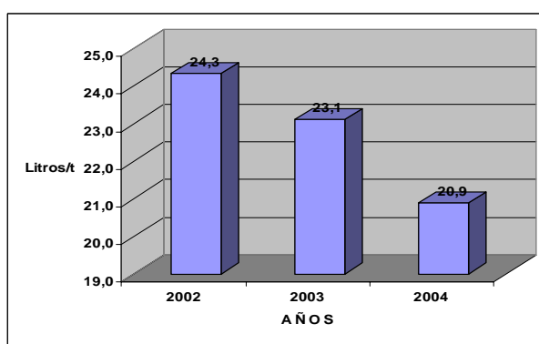
Gráfico 5. Consumo de diesel
