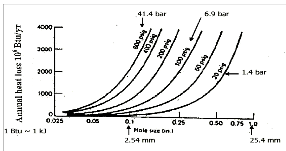
Gráfico 6. Determinación de pérdidas de vapor a diferentes presiones manométricas y diámetros del orificio de fuga.
